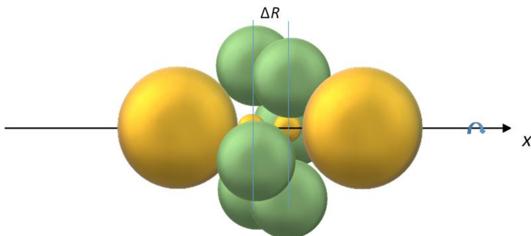
Fig. 11. The interval \Delta R between the 2p -electrons of the semi-closed parts of the subshell Рис. 11. Интервал \Delta R между 2p -электронами полузакрытых частей подоболочки
